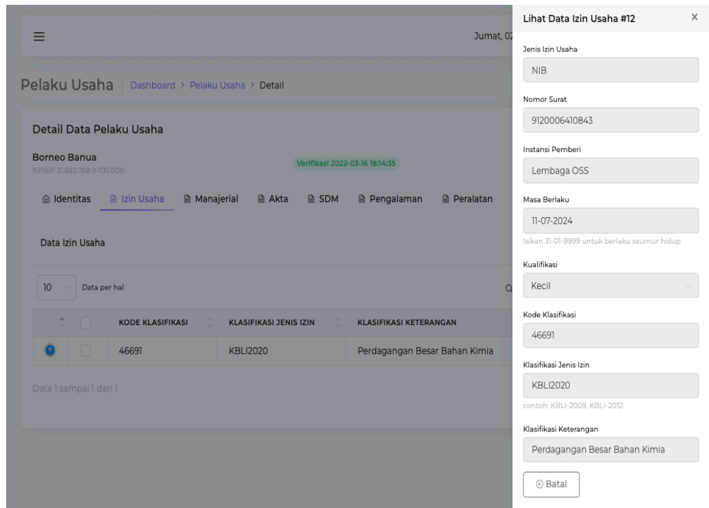
Gambar 13 Melihat Data
