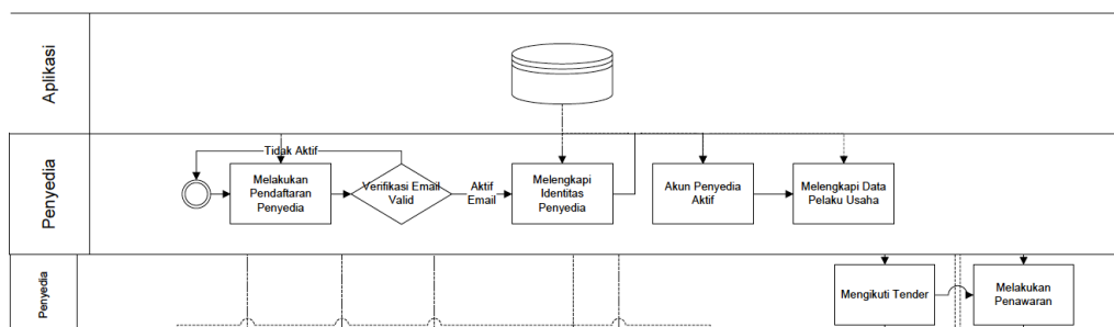
Gambar 17 Alur Penyedia
