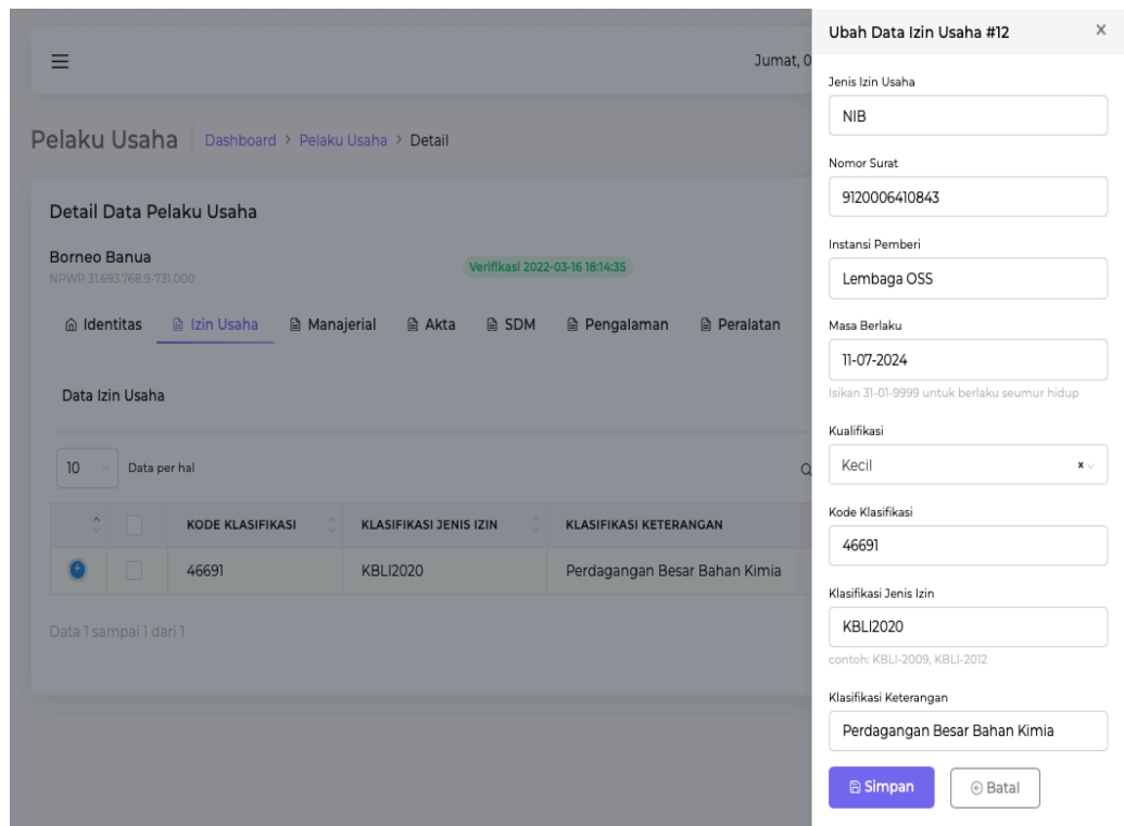
Gambar 14 Ubah Data
