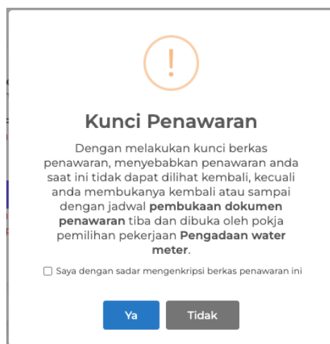
Gambar 43 Kunci Penawaran
